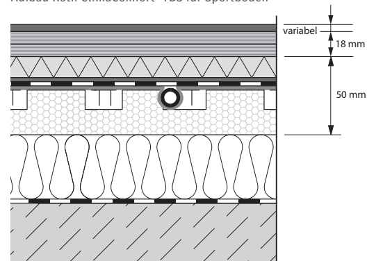
Aufbau Roth KlimaComfort® TBS für Sportböden
