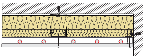
Wandaufbau Roth ClimaComfort® Panel
