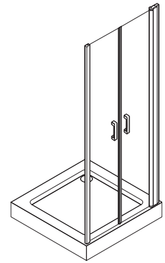
Niche door 2 × CP245 (width 900 mm)
