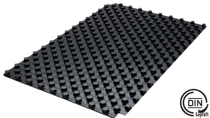
Roth Noppenfolie 14-16 mm (ohne Dämmung), zur Verlegung auf bauseitiger Dämmung
