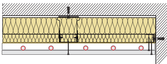
Wandaufbau Roth ClimaComfort® Panel
