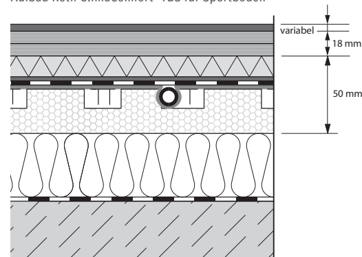
Aufbau Roth ClimaComfort® TBS für Sportböden
