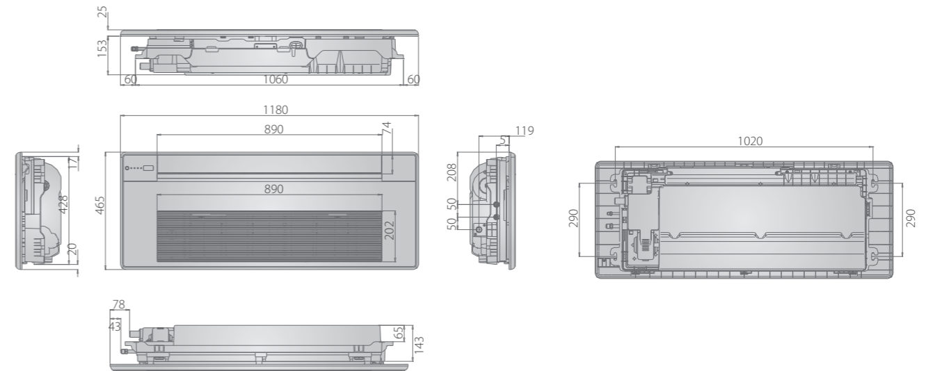
MKC-V300R-B
