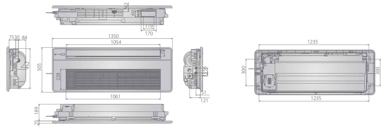
MKC-V400R-B MKC-V600R-B
